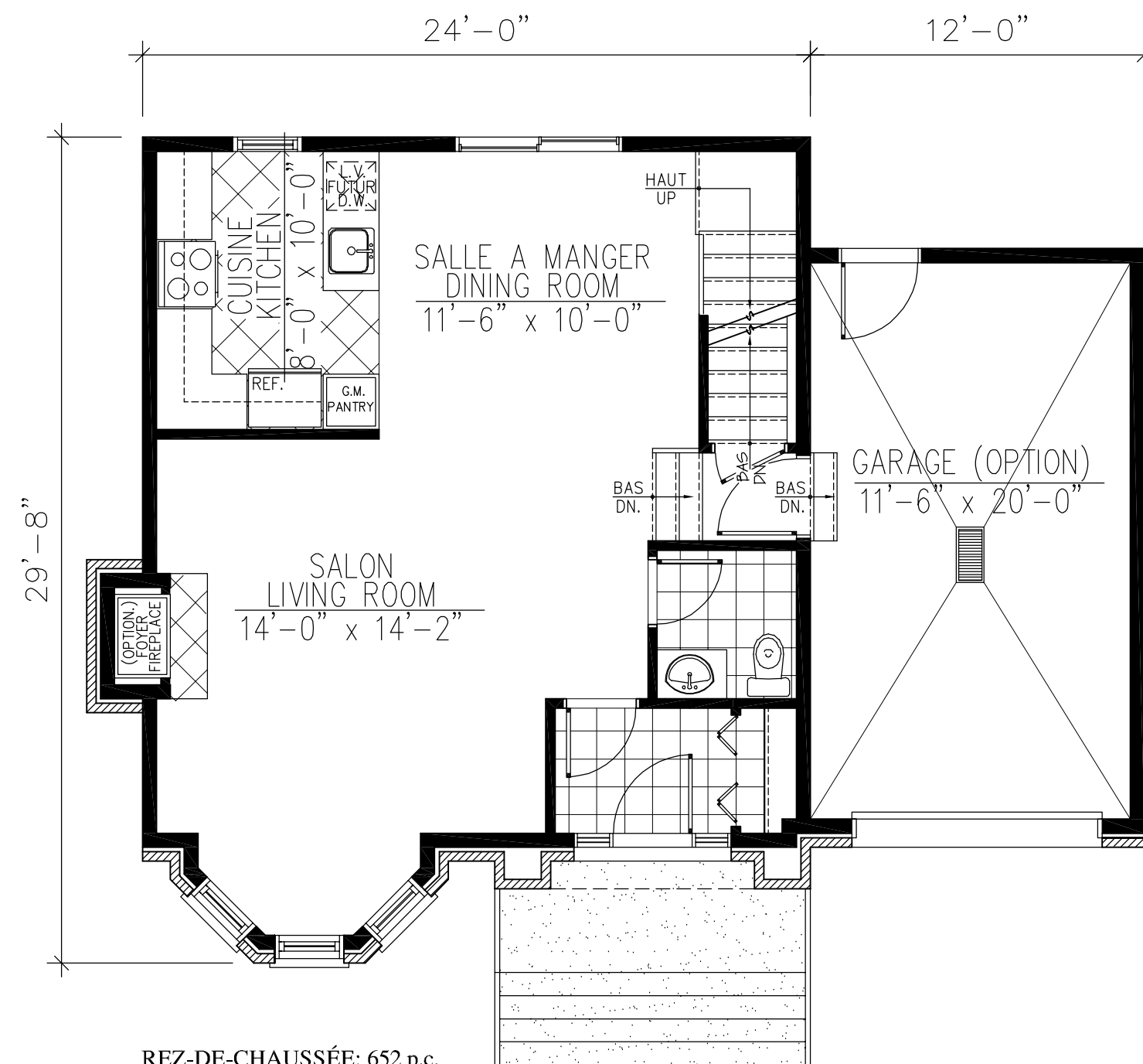
no.656 REZ-DE-CHAUSSÉE: 652 p.c. MAIN FLOOR: 652 sq.ft.
