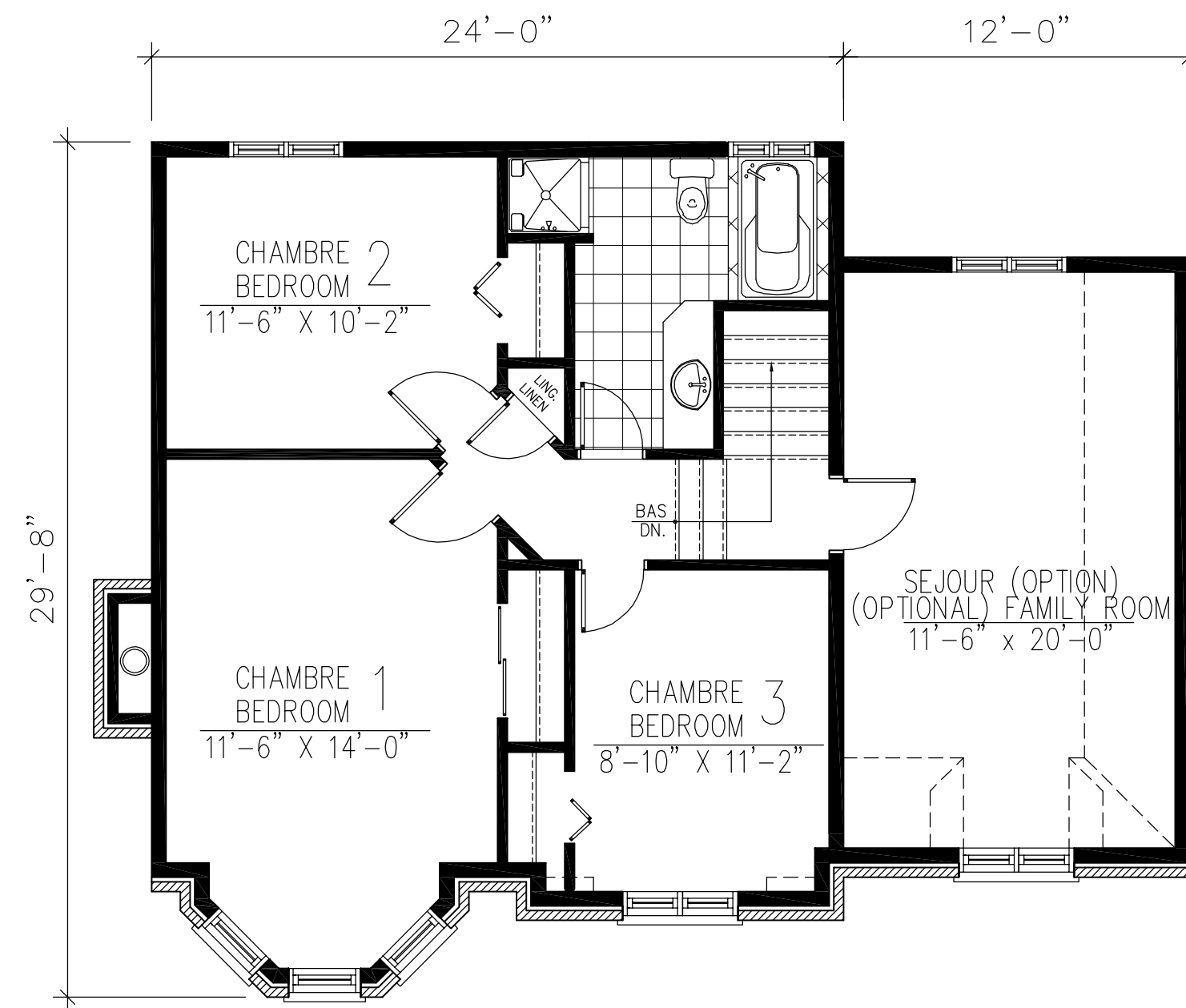
ÉTAGE: 663 p.c. SECOND FLOOR: 663 sq.ft.
